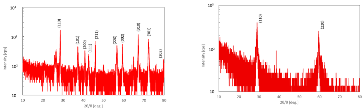
図 2 X 線回折方による粉末状試料のプロファイル(左)と、結晶のファセット面のプロファイル
